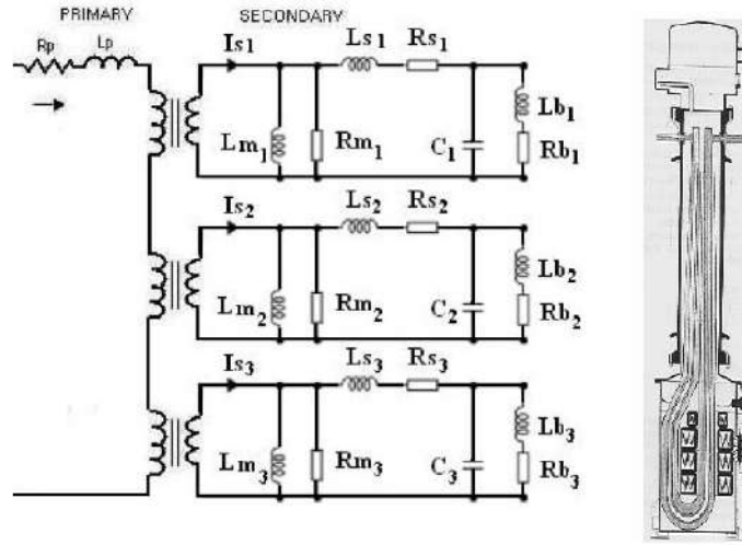
Şekil 2: Yüksek Frekanslı Akım Trafosu Eşdeğer devresi
